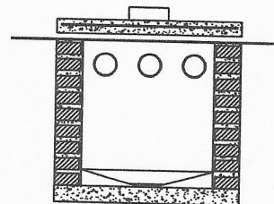
CORTE - BB
