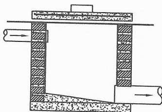
CORTE - AA
