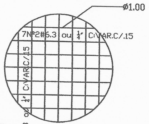
ARMAÇÃO DA TAMPA
