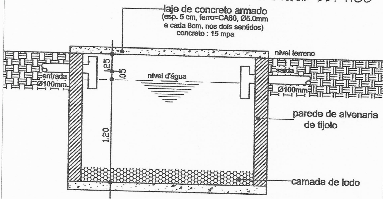
CORTE - AB
