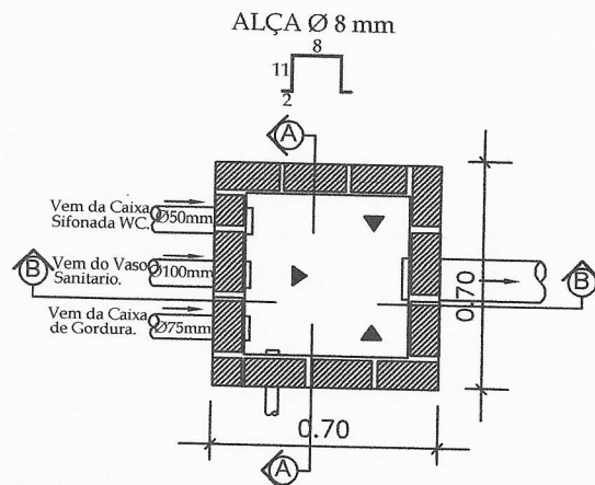
PLANTA BAIXA
